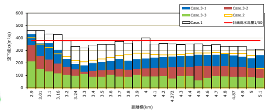
図2 香川県高瀬川における UAV を用いた地形測量結果とそれを用いた流下能力評価結果
